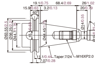
DIN40
