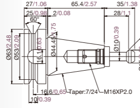
BT40
