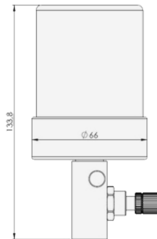
干油型
