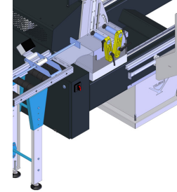
Short cut system Kısa profil kesme sistemi
