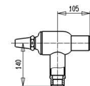
EA40-VA/G1"-II (inklusive G1" Gewinde-Anschluss)
