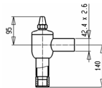
EA32/G1"-I (inklusive G1" Gewinde-Anschluss)
